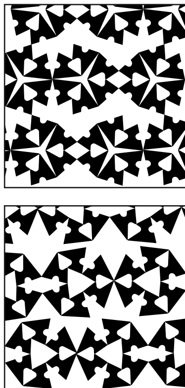
Комбинаторика
