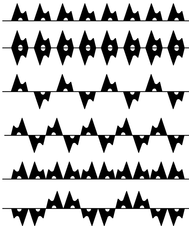
Комбинаторика
